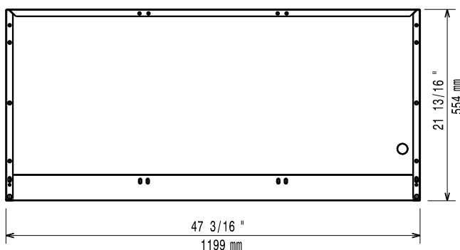
Boven aanzicht
